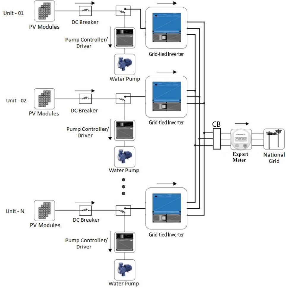
চিত্র-৪: একাধিক ইনভার্টার ব্যবহার করে সংযোগ প্রক্রিয়া
